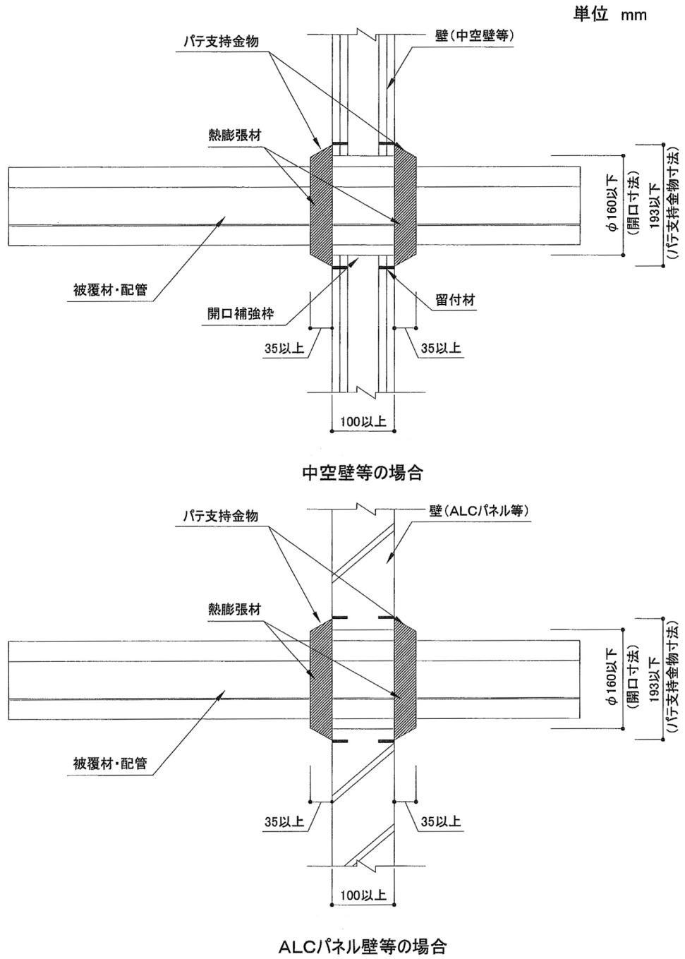
図-1 標準施工図
