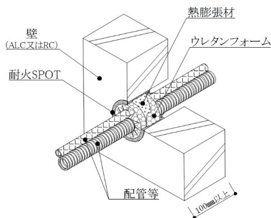
図-2 壁施工完成図 (ALC・RC 壁)
