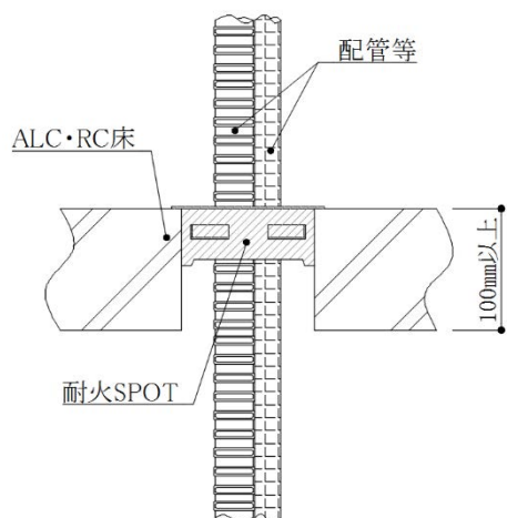
図-1 床施工完成図 (ALC・RC 床)
