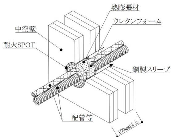
図-3 中空壁施工完成図
