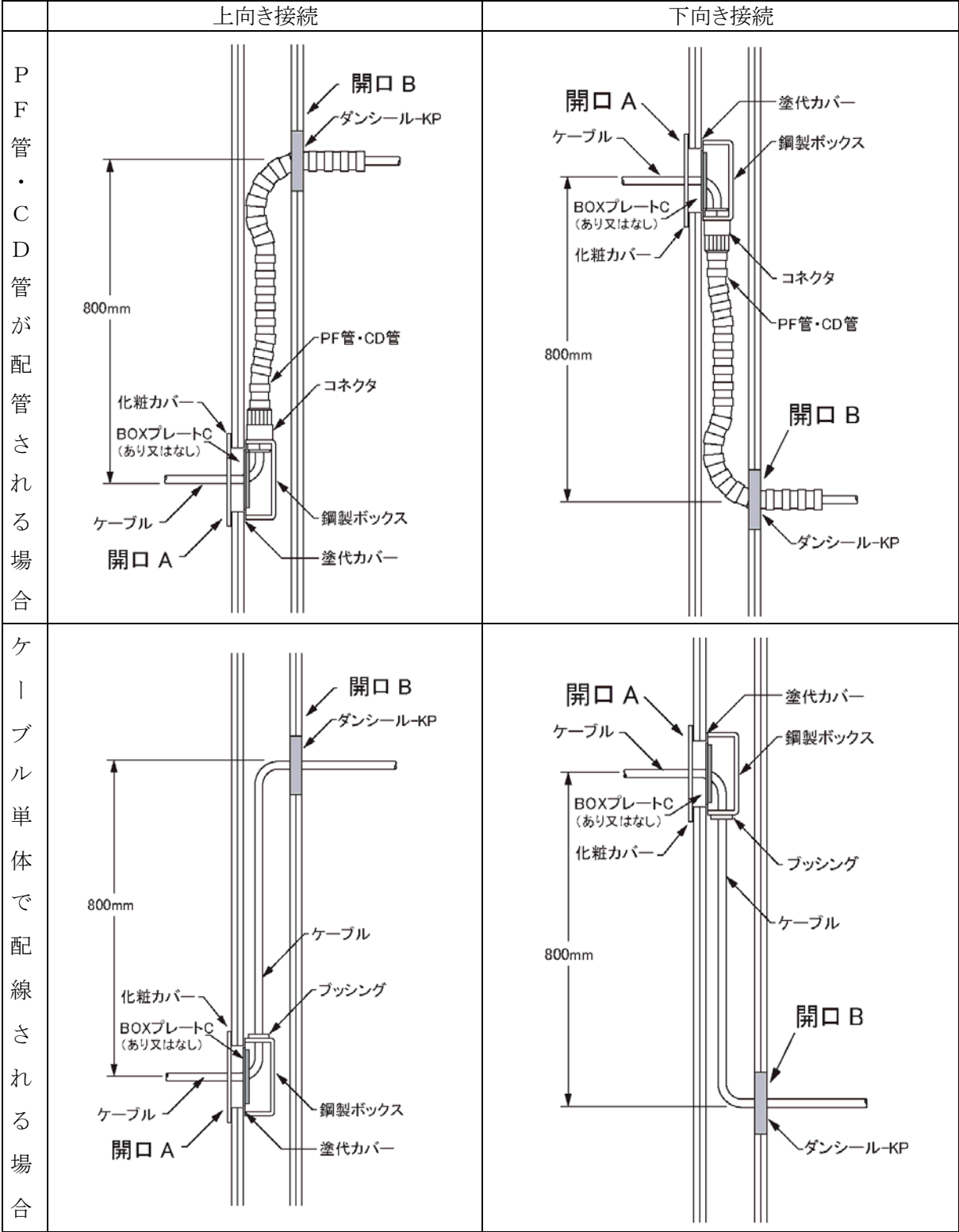
図1 標準施工図
