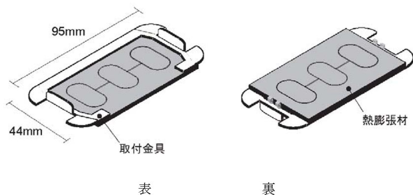
図 2 BOX プレート C
