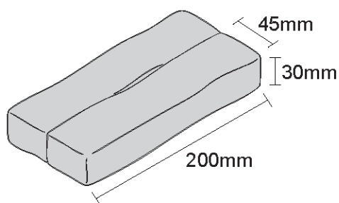
図 3 ダンシール-KP(別売)
